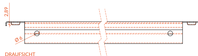
DRAUFSICHT
