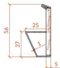
SEITENANSICHT
