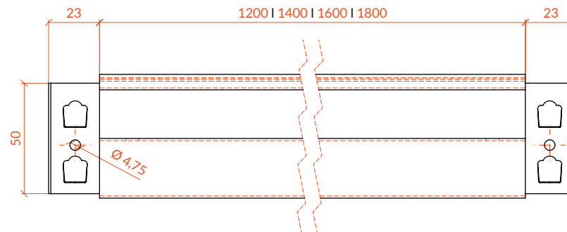
VORDERANSICHT
