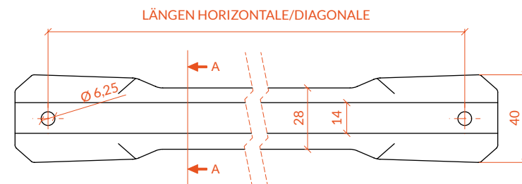
VORDERANSICHT
